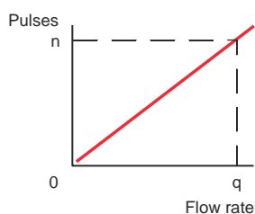
Linear pulses
