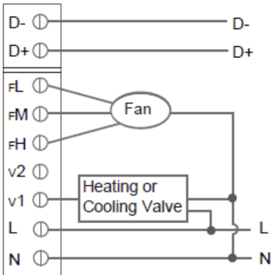
Fig. 2. Honeywell Home VC4013/VN4013/VS4016 Wiring
