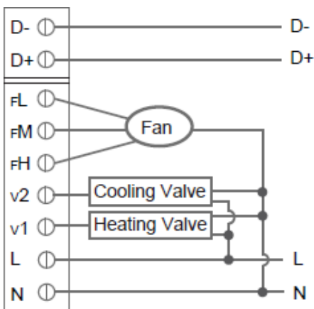
Fig. 4. Honeywell Home VC4013/VN4013/VS4016 Wiring
